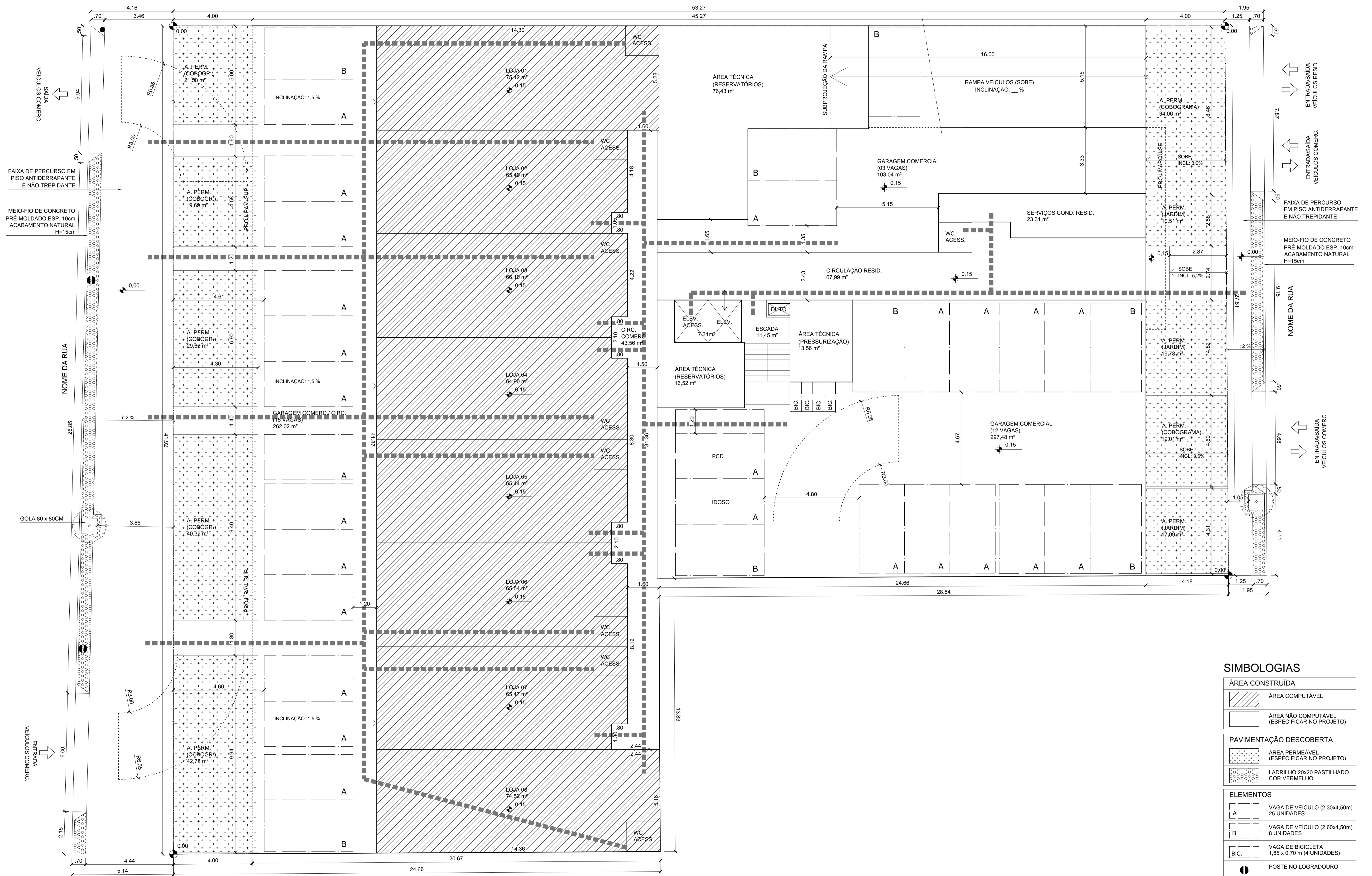
PLANTA 1º PAVIMENTO ESC.: 1/100
